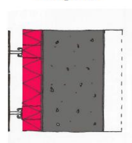
materiales composite
